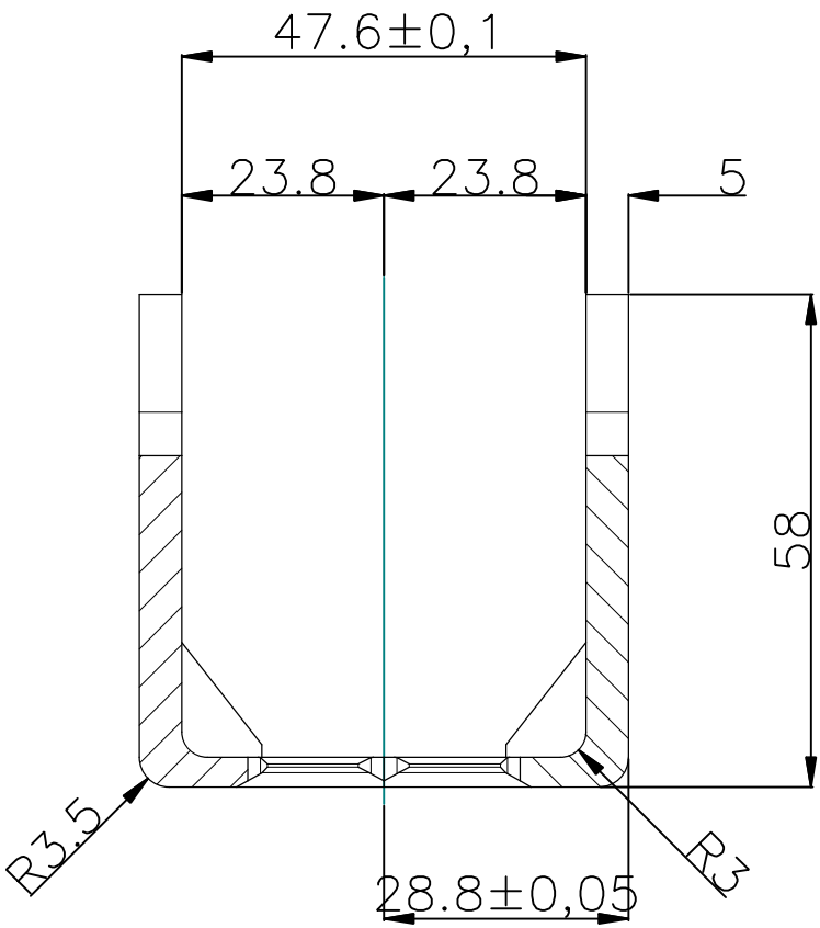
PREREZ A-A
